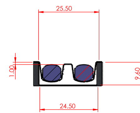
SECTION N-N SCALE 1 : 1
